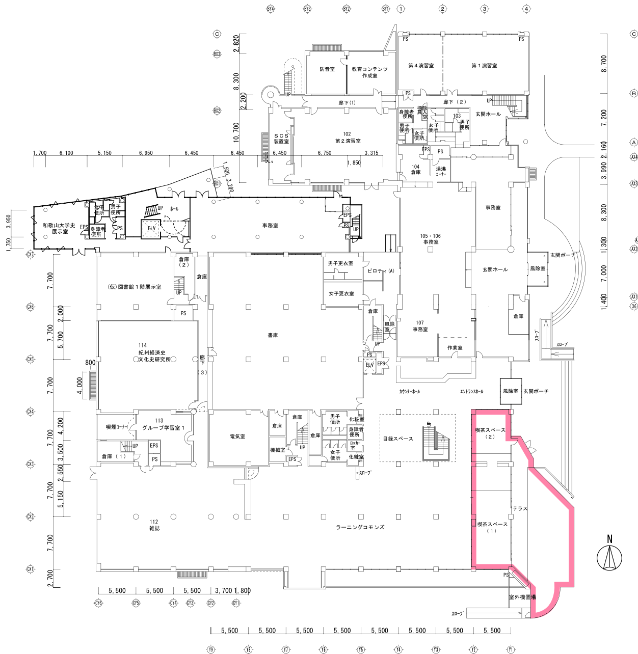
1階平面図 S=1/400
